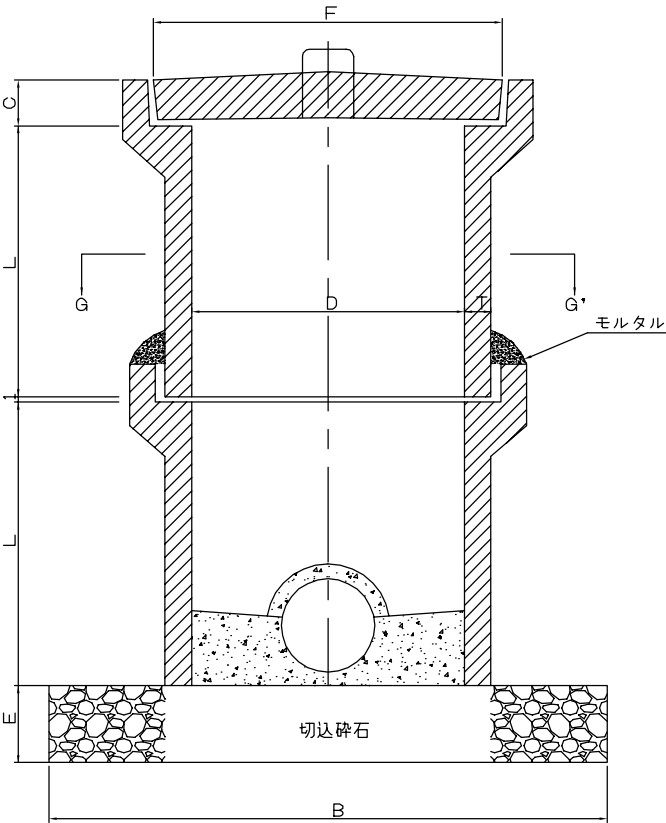
縦断面図
