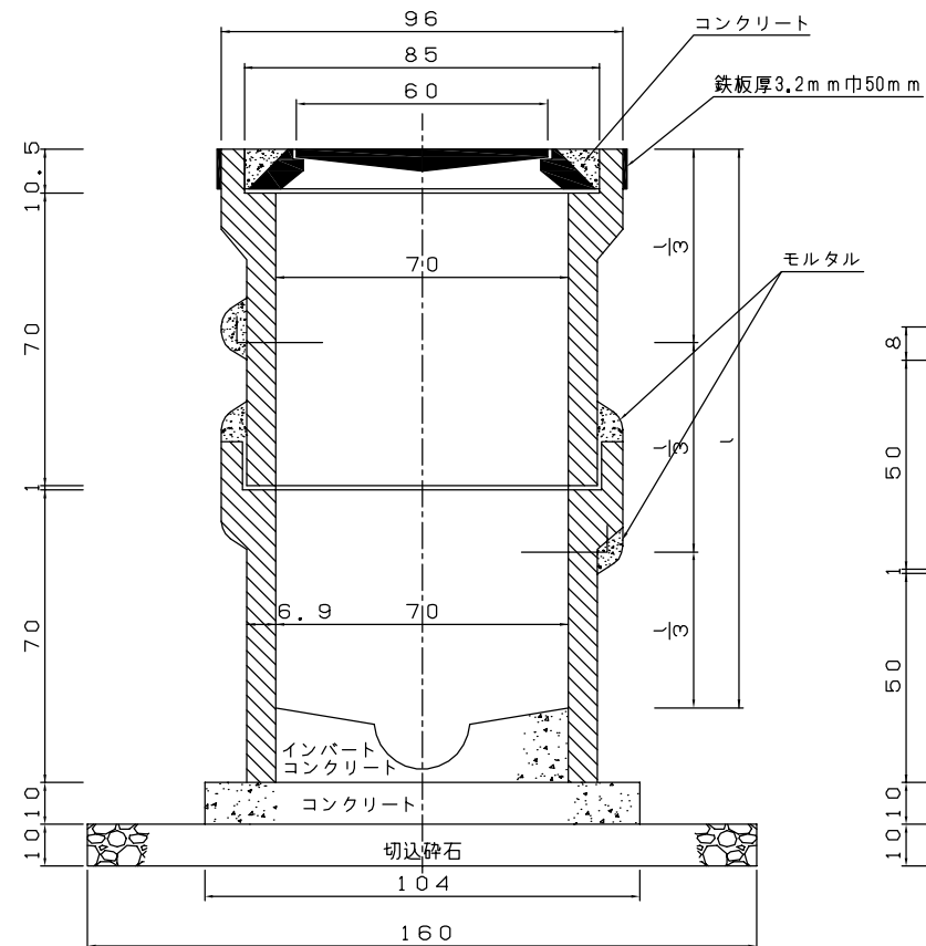
断面図
