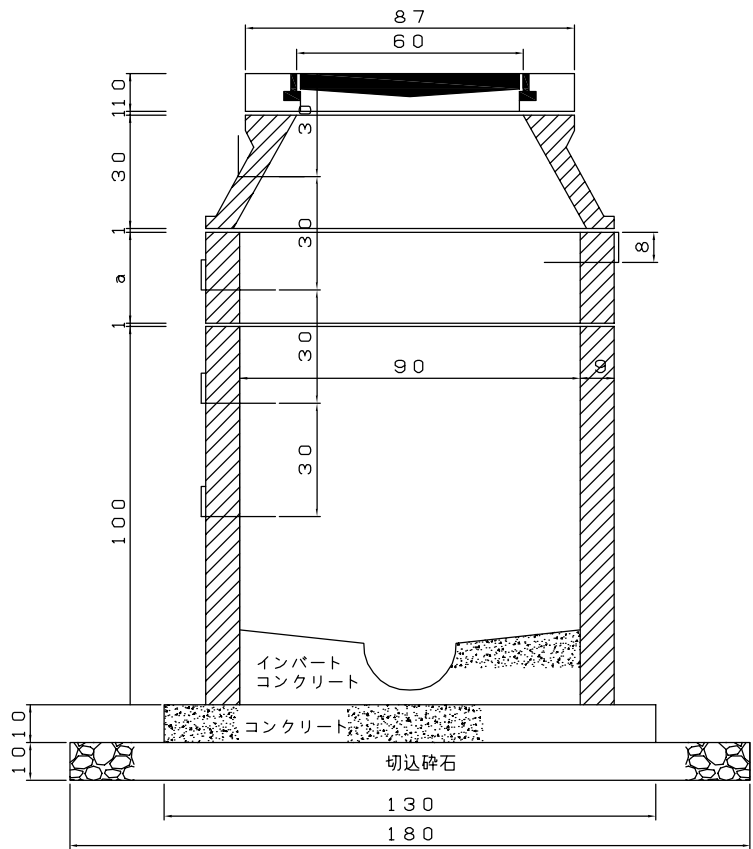
断面図
