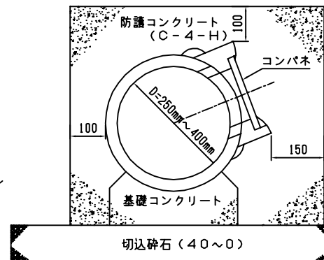
コンクリートソケット使用の場合
