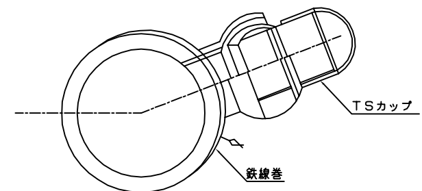
塩ビ自在ソケット使用の場合
