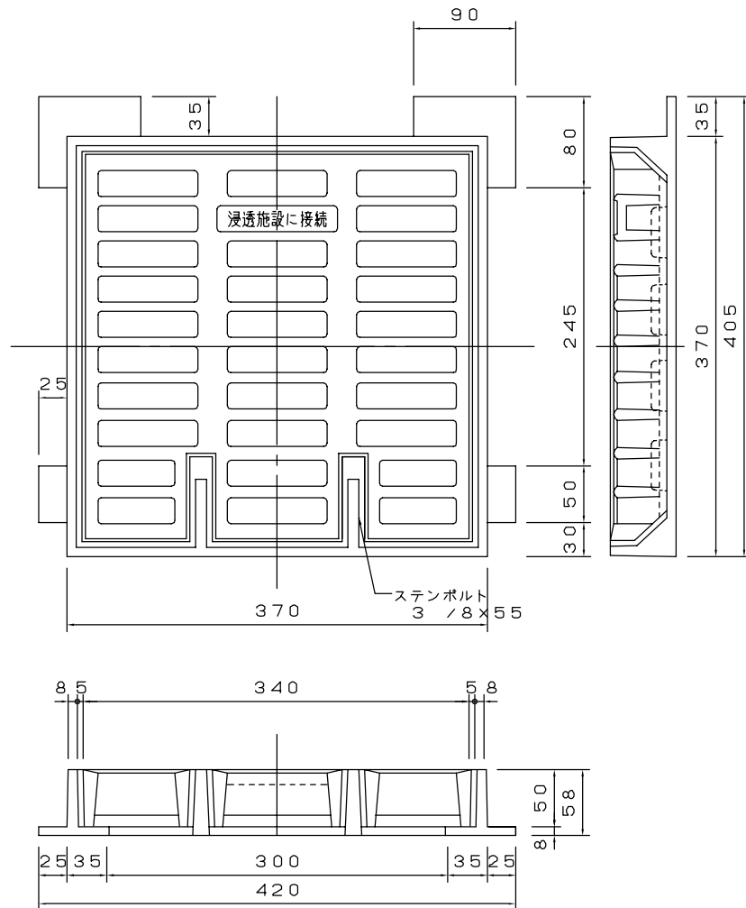
ダクタイトル蓋（２型雨水枳用）改良型
