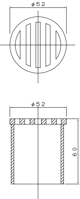
空気孔詳細図
