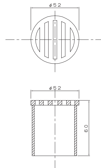
空気孔詳細図
