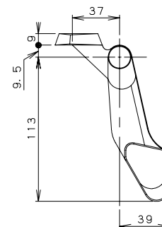
⑤ 多機能錠詳細図
