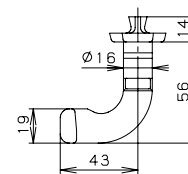
⑥ ロック金具詳細図
