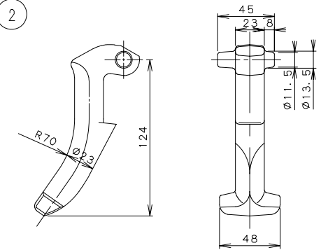
③ 蝶番詳細図
