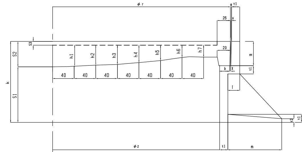
寸法
