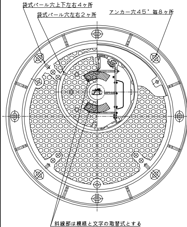
流雪溝送水管用マンホール鉄蓋
