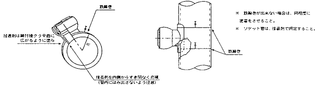
図7-5 支管の接合
