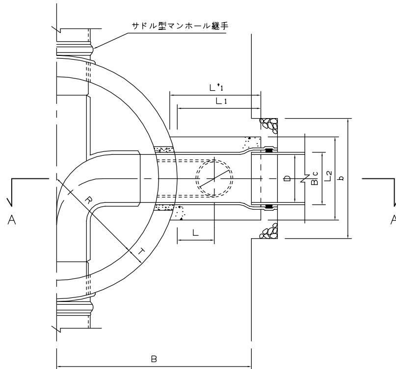
平 面 図
