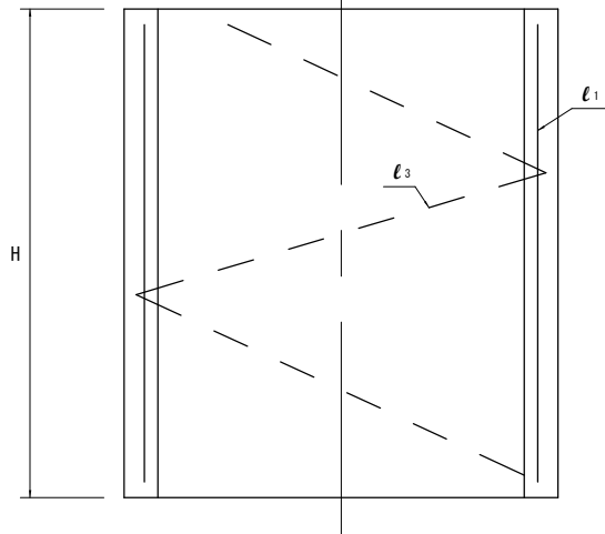
(断面図)
