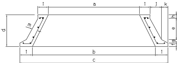
(断面図)
