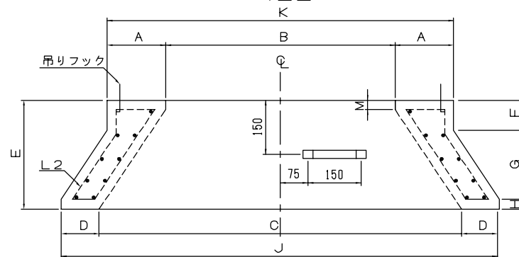
(断面図)
