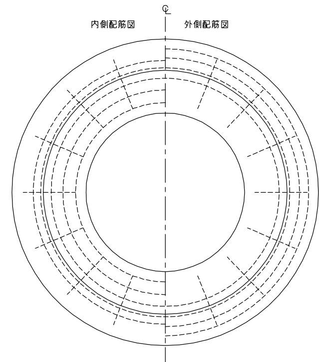
(平面図)
