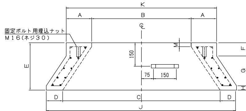
（断面図）
