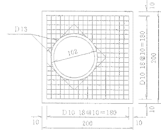
＜頂版配筋図＞ S=1/50
