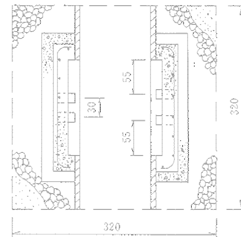
＜平面図＞ S=1/60
