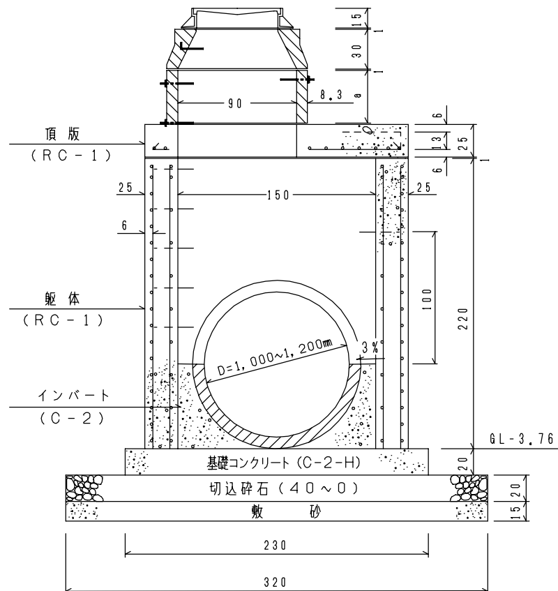
< 断 面 図 > S=1/40
