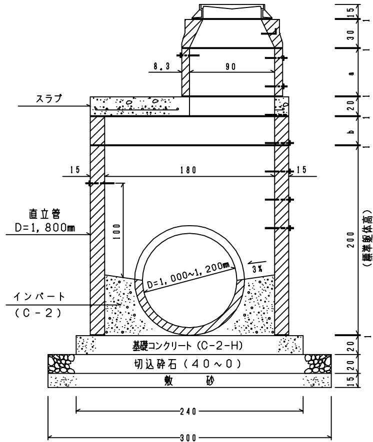
< 断面図 > S=1/40
