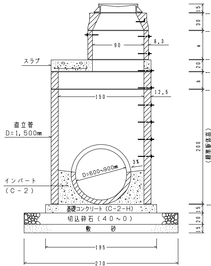
< 断面図 > S=1/40
