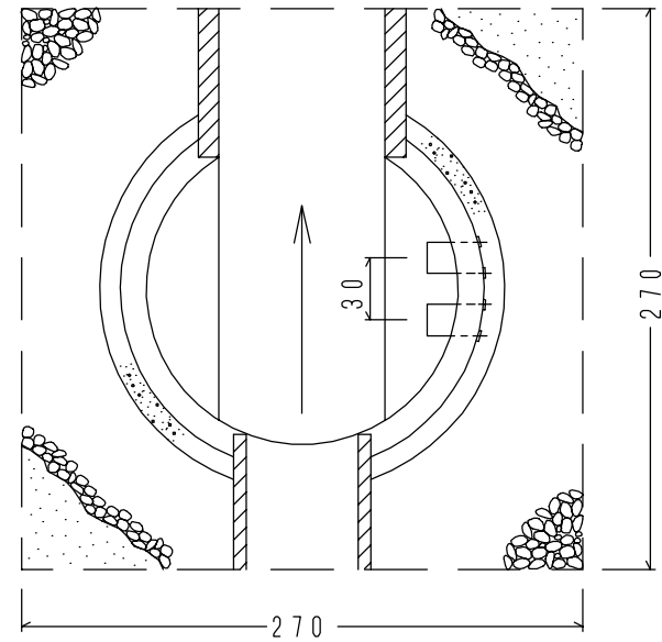
< 平面図 > S=1/60
