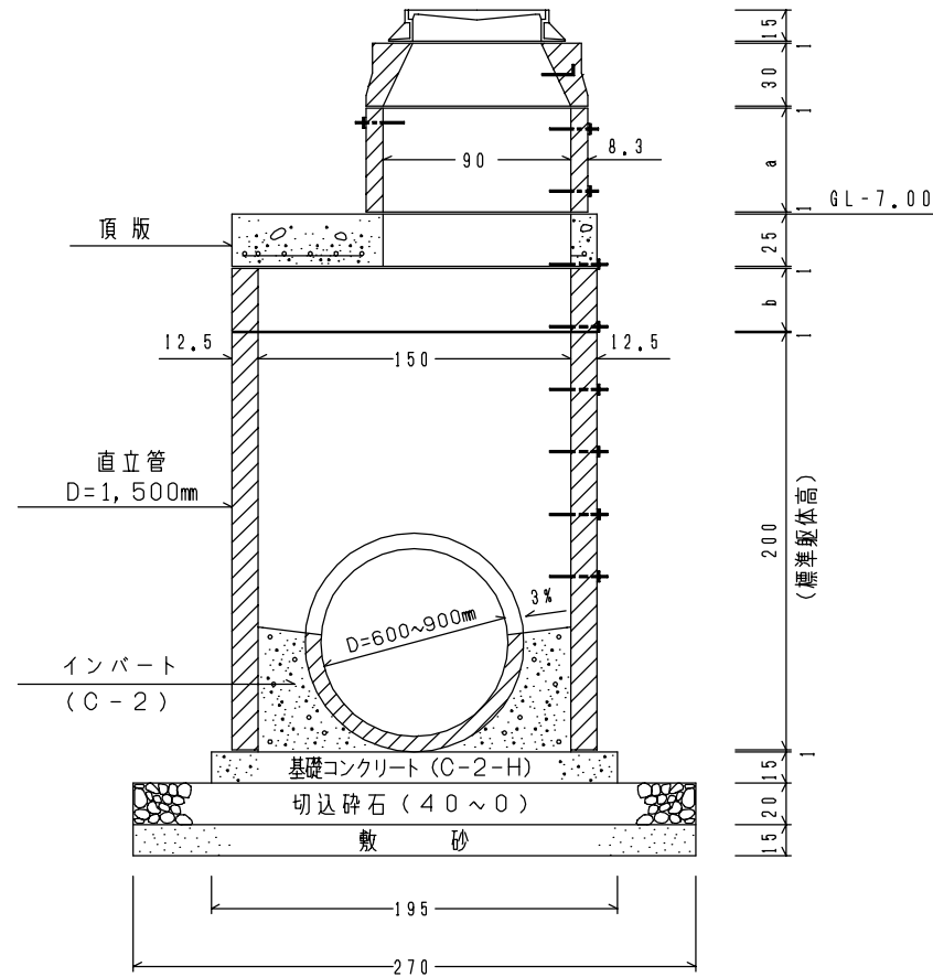
< 断面図 > S=1/40
