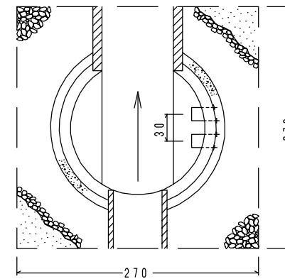
< 平面図 > S=1/60
