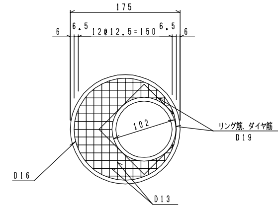
< 頂版配筋図 > S=1/60
