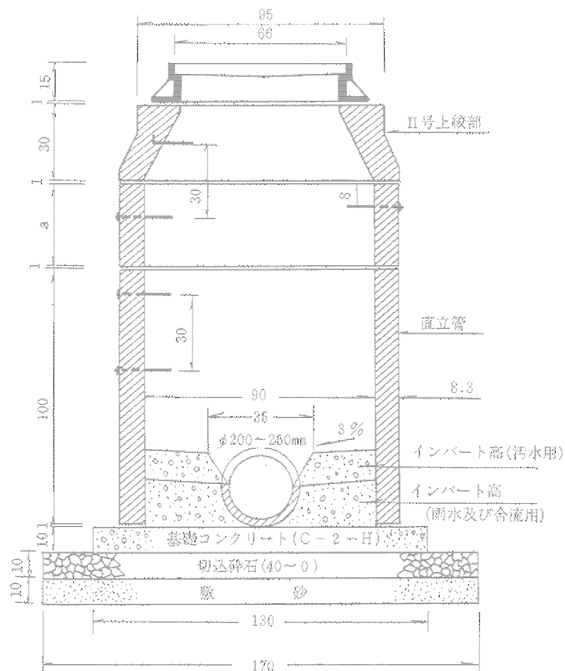
〈断面図〉 S=1/20
