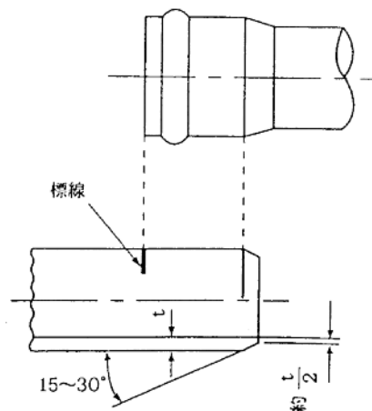
図 5-2 面取り標線
