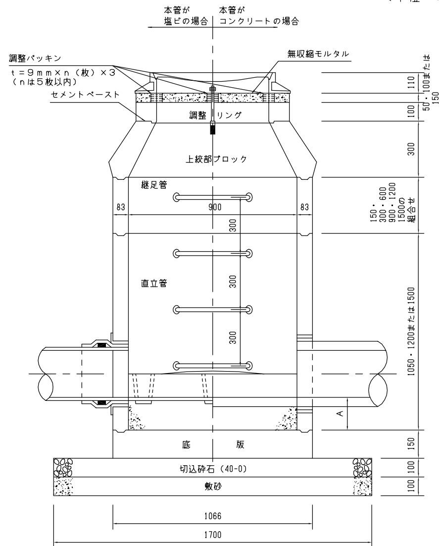
A-A' S=1/20
