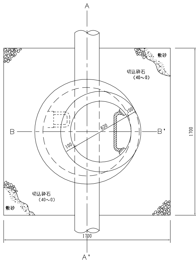
平面図 S=1/20
