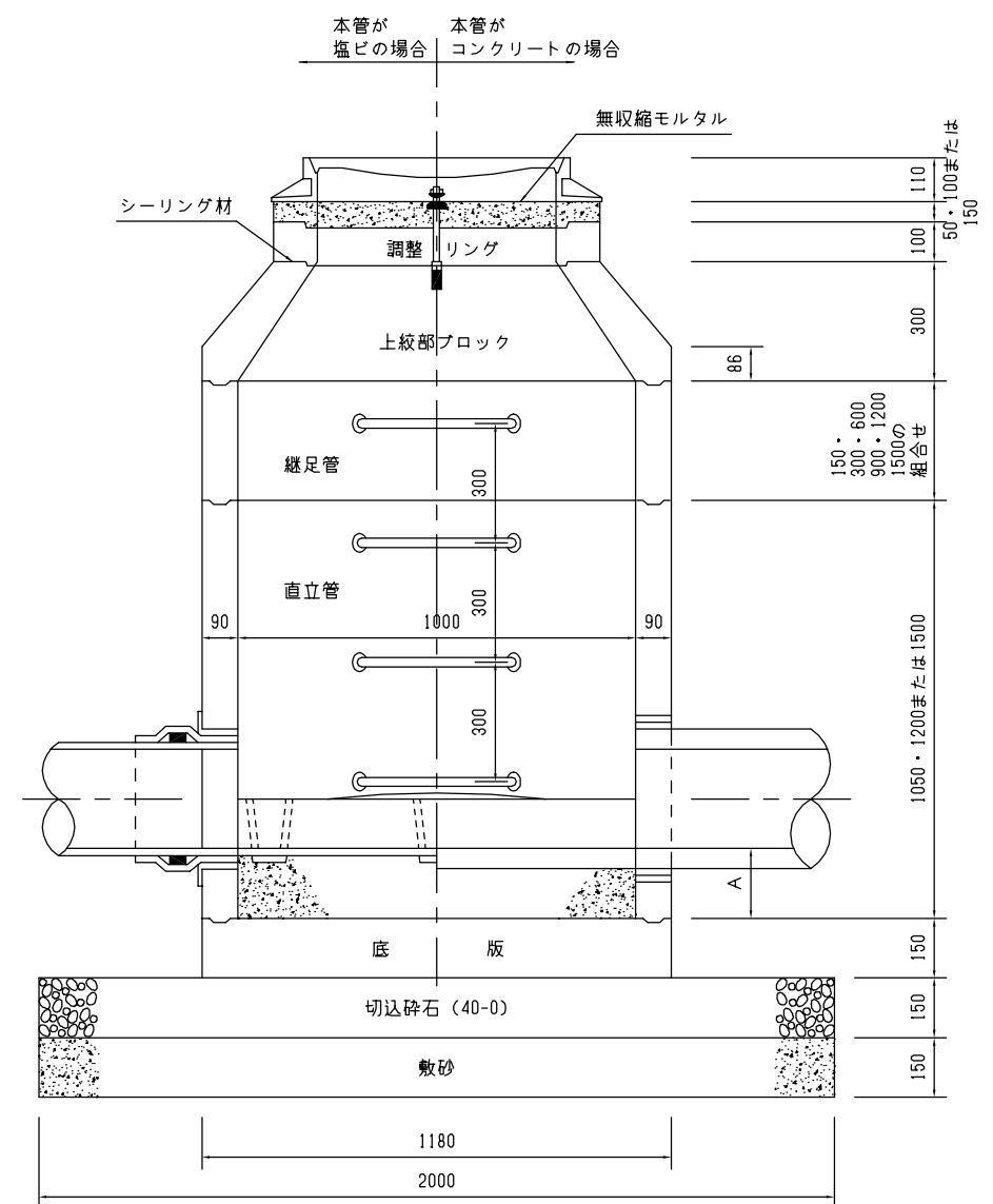
A-A' S=1/20
