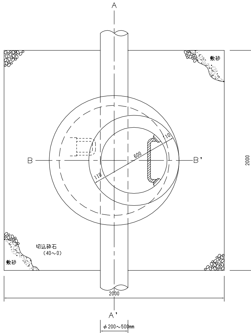
平面図 S=1/20
