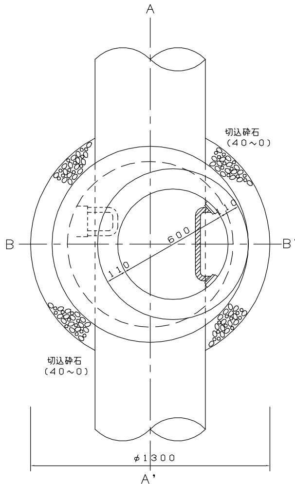
平面図 S=1/20
