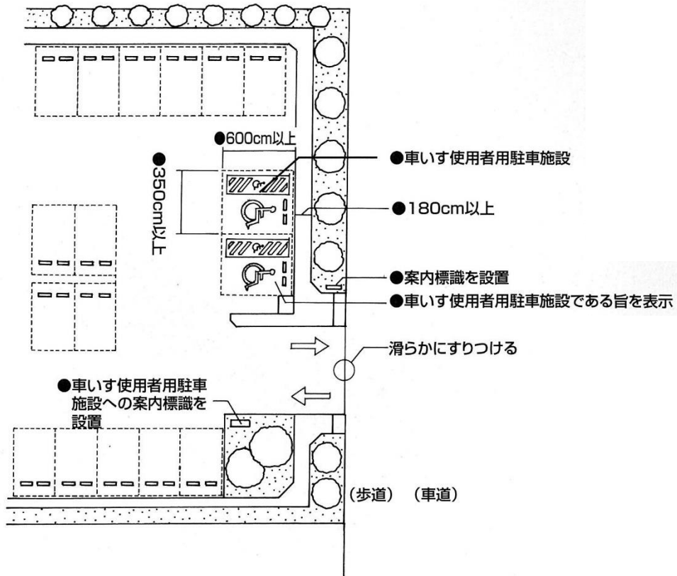
■ 車いす使用者用駐車施設の標識の例
