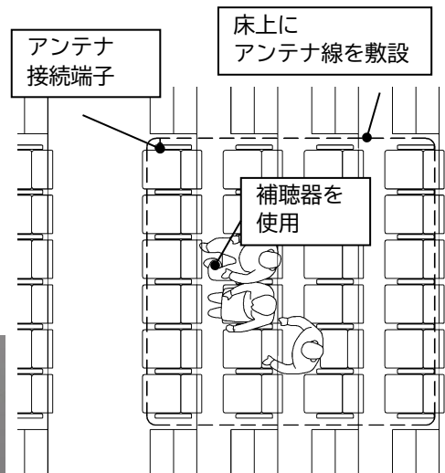
・難聴者の補聴器に雑音の少ないクリアな音声を届けることができるヒアリングループ(磁気ループ)システム(写真と図は、床上に設置するタイプ)
