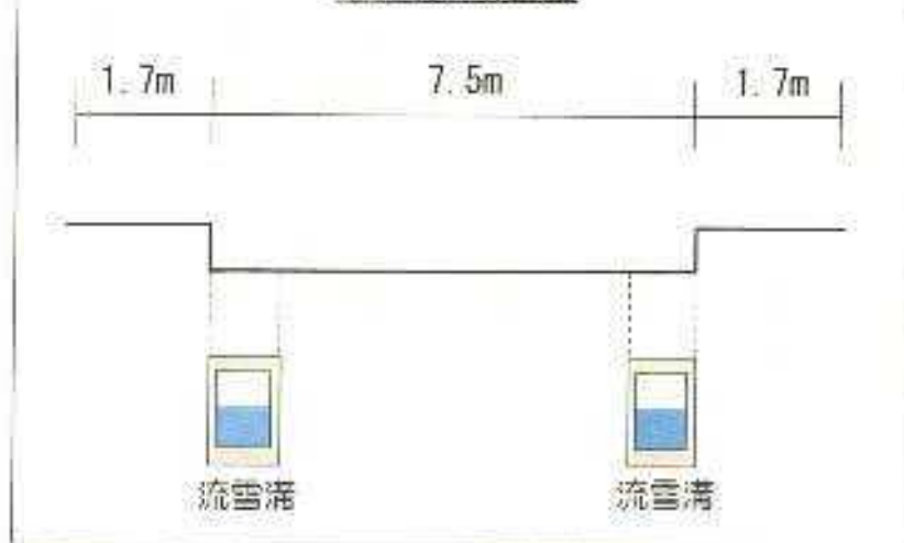
稲荷線 断面図
