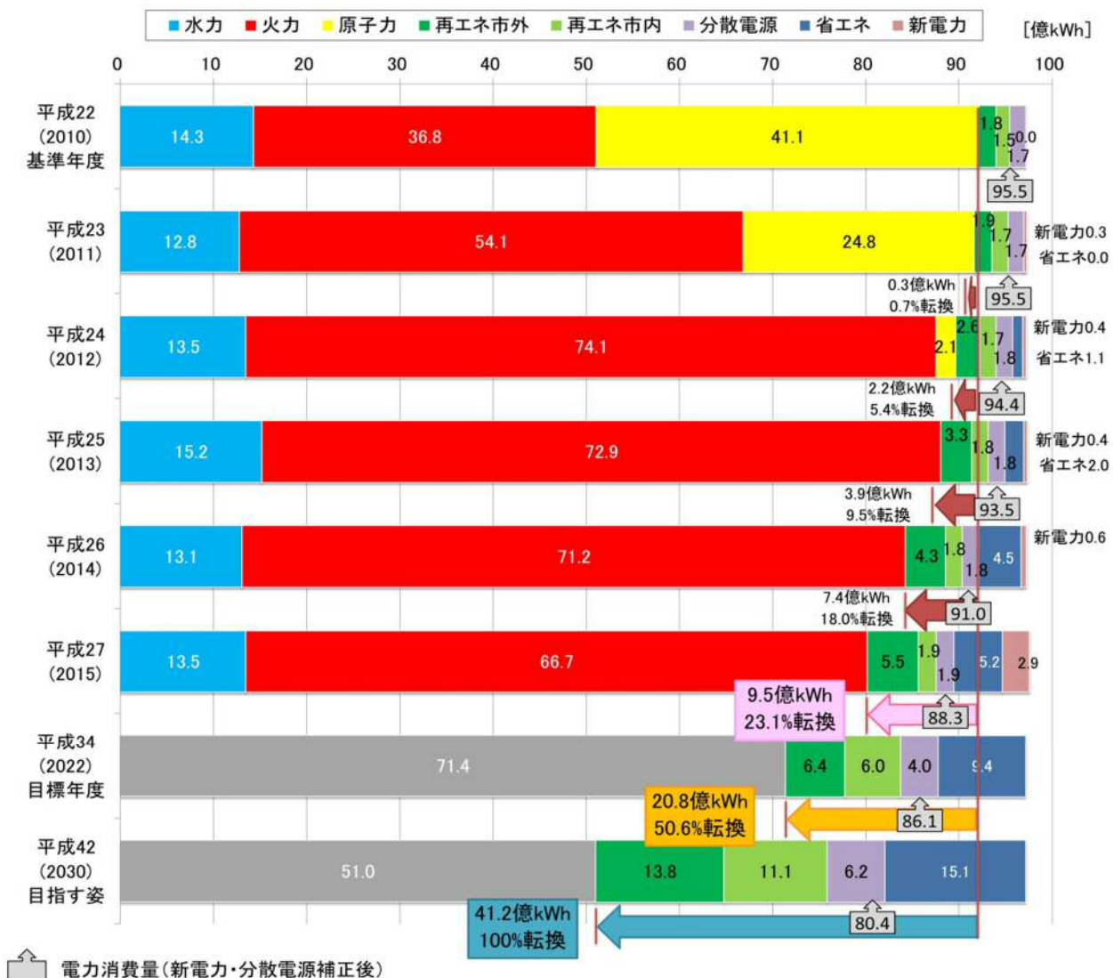
図6 エネルギー転換の達成状況
