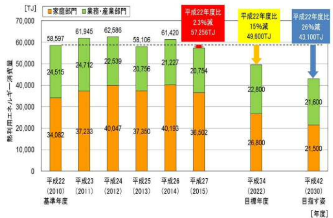
図2 熱利用エネルギー消費量の達成状況
