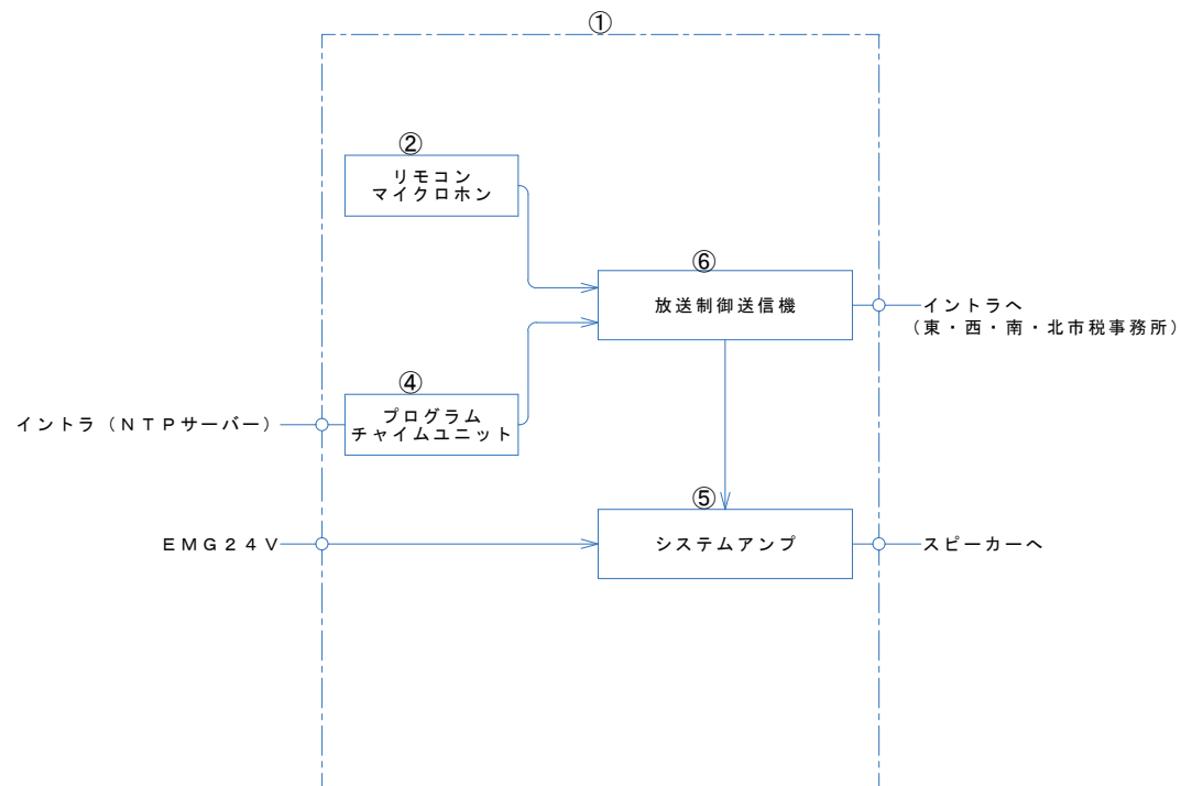
ブロック図
