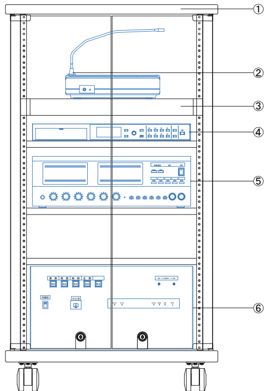
機器収納庫姿図
