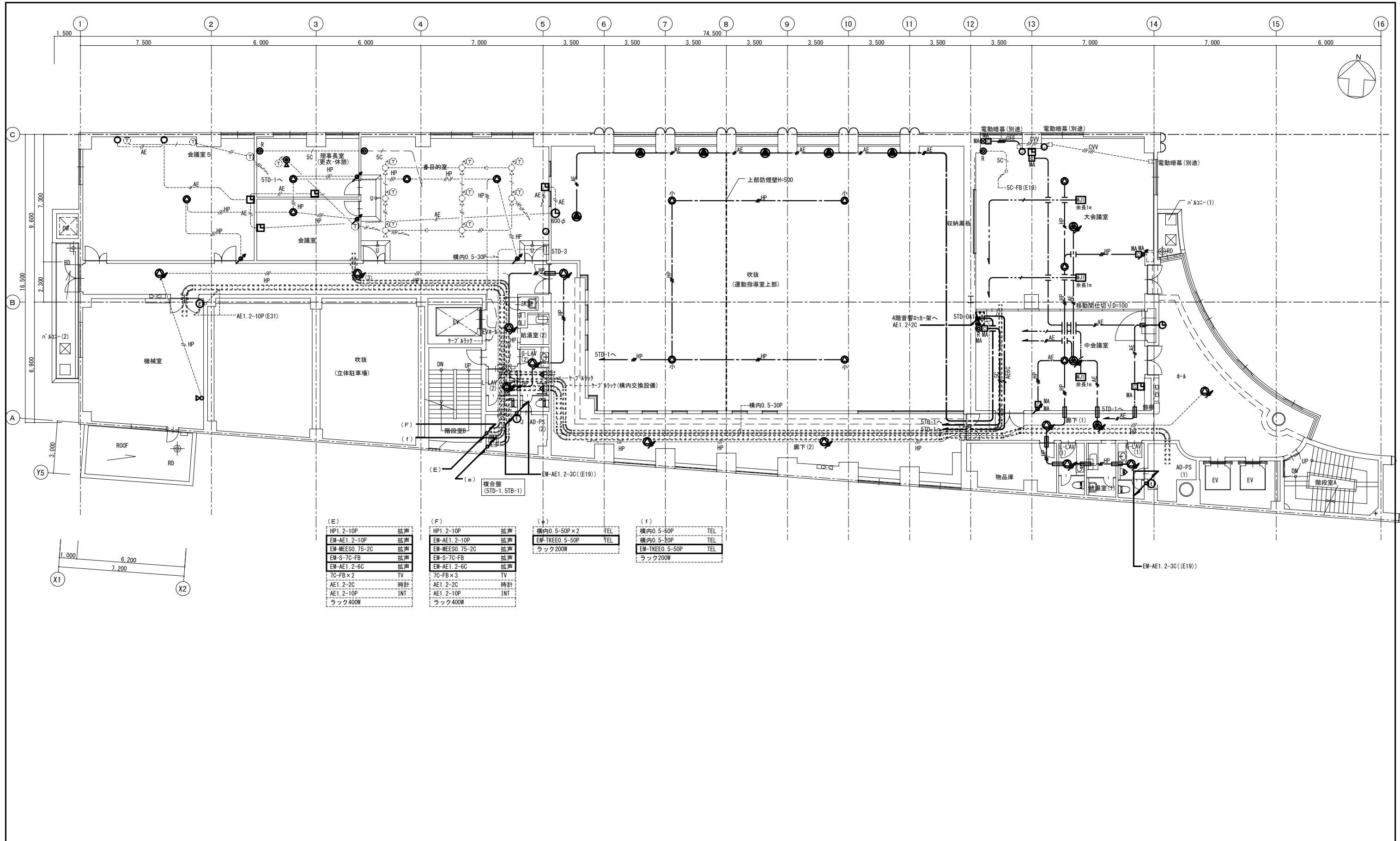
弱電設備 5階平面図 (改修) A1=1/100 ※細線が既設、太線が改修
