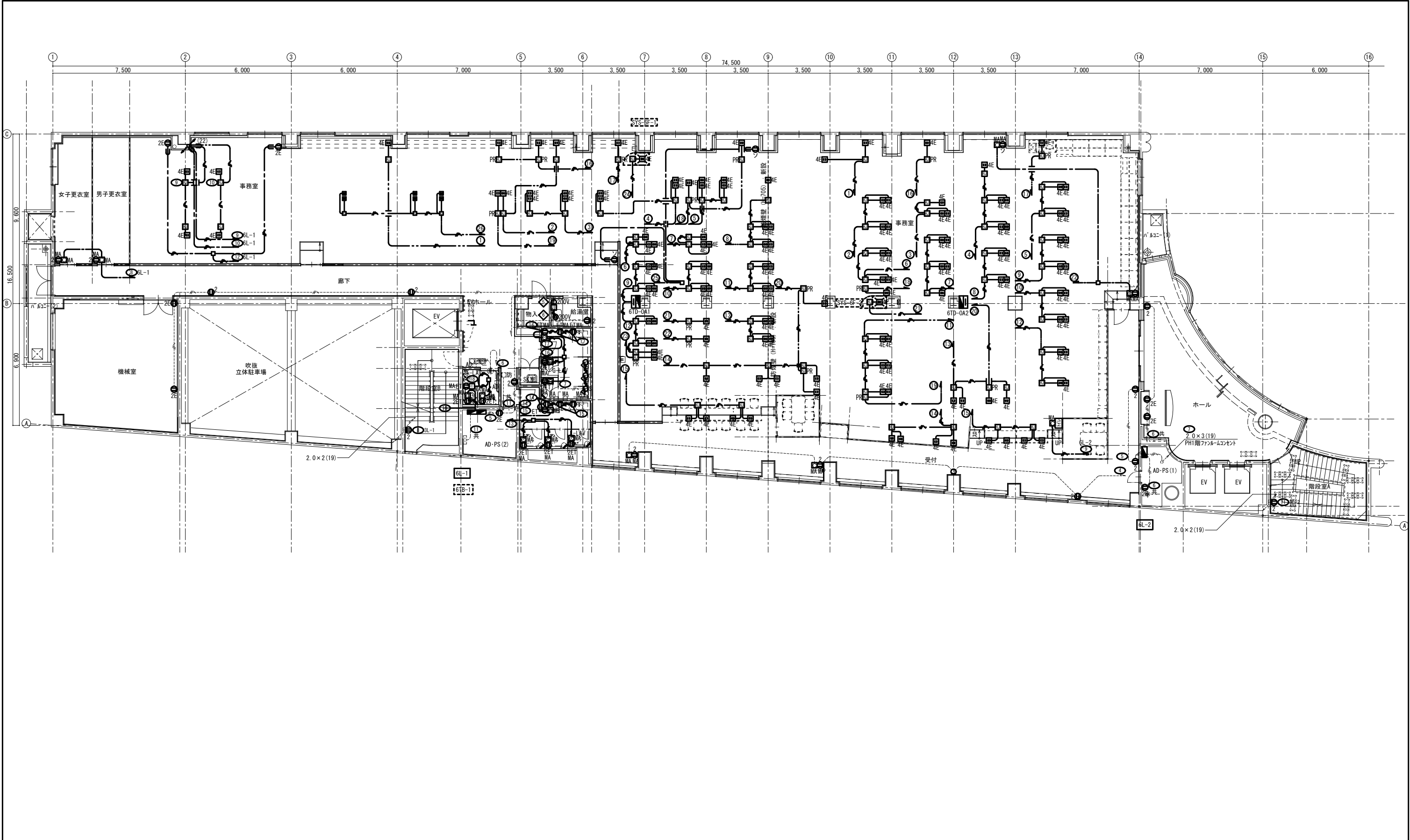
コンセント設備 6階平面図 (改修) A1=1/100 ※細線が既設、太線が改修
