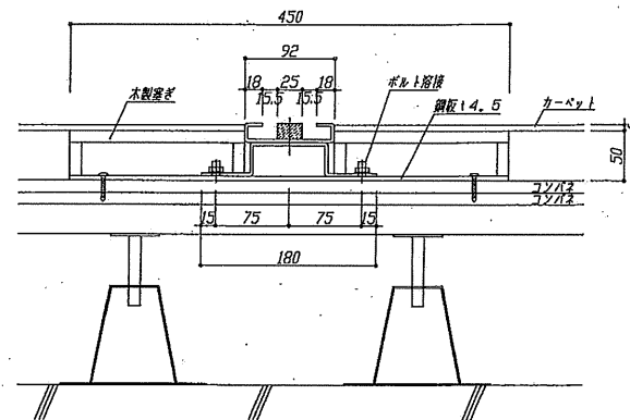
＜レール断面図＞
