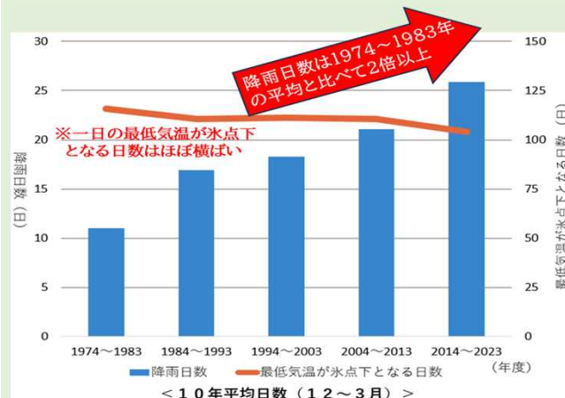
積雪寒冷地特有の舗装損傷
