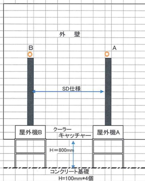
立面図
