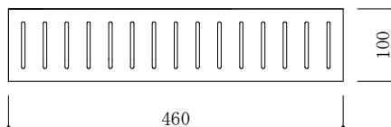
包丁受け 詳細図
