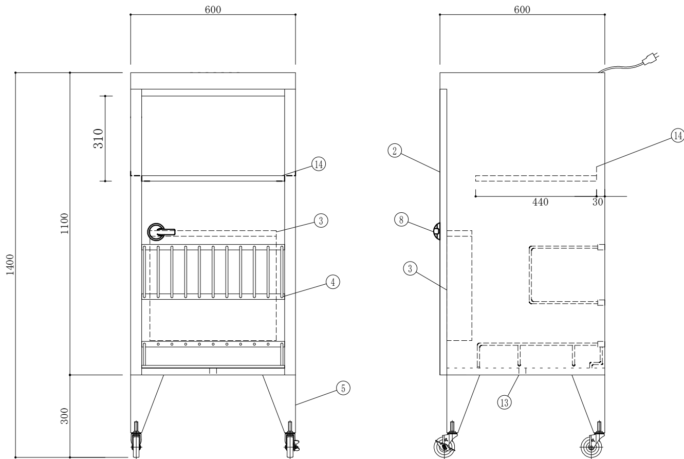
包丁受け 詳細図
