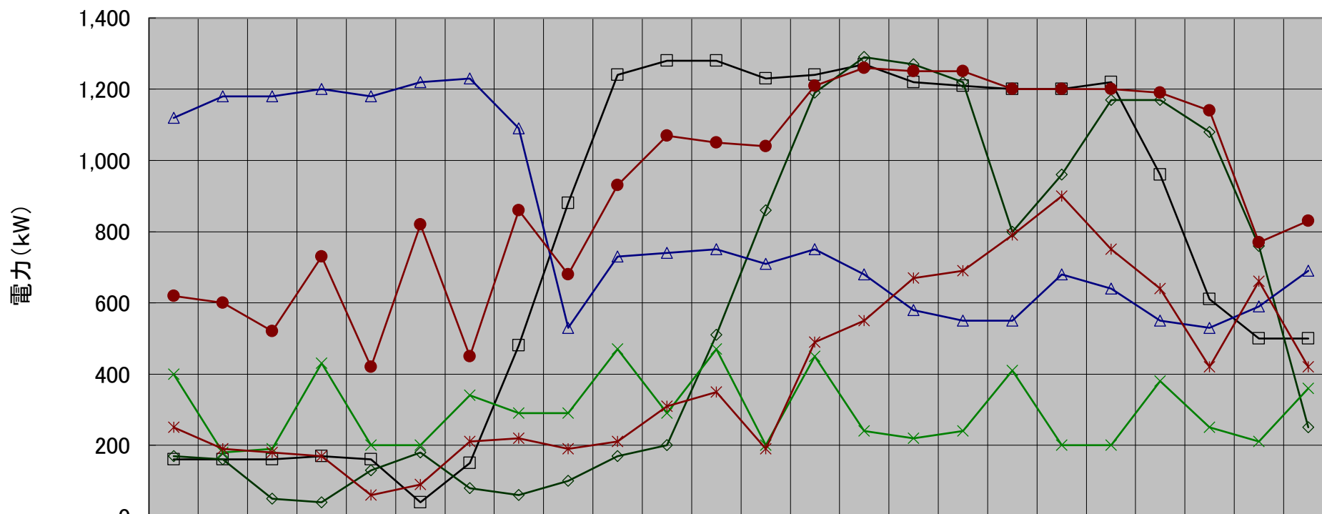
月別最大負荷日ロードカーブ(令和4年度下期)
