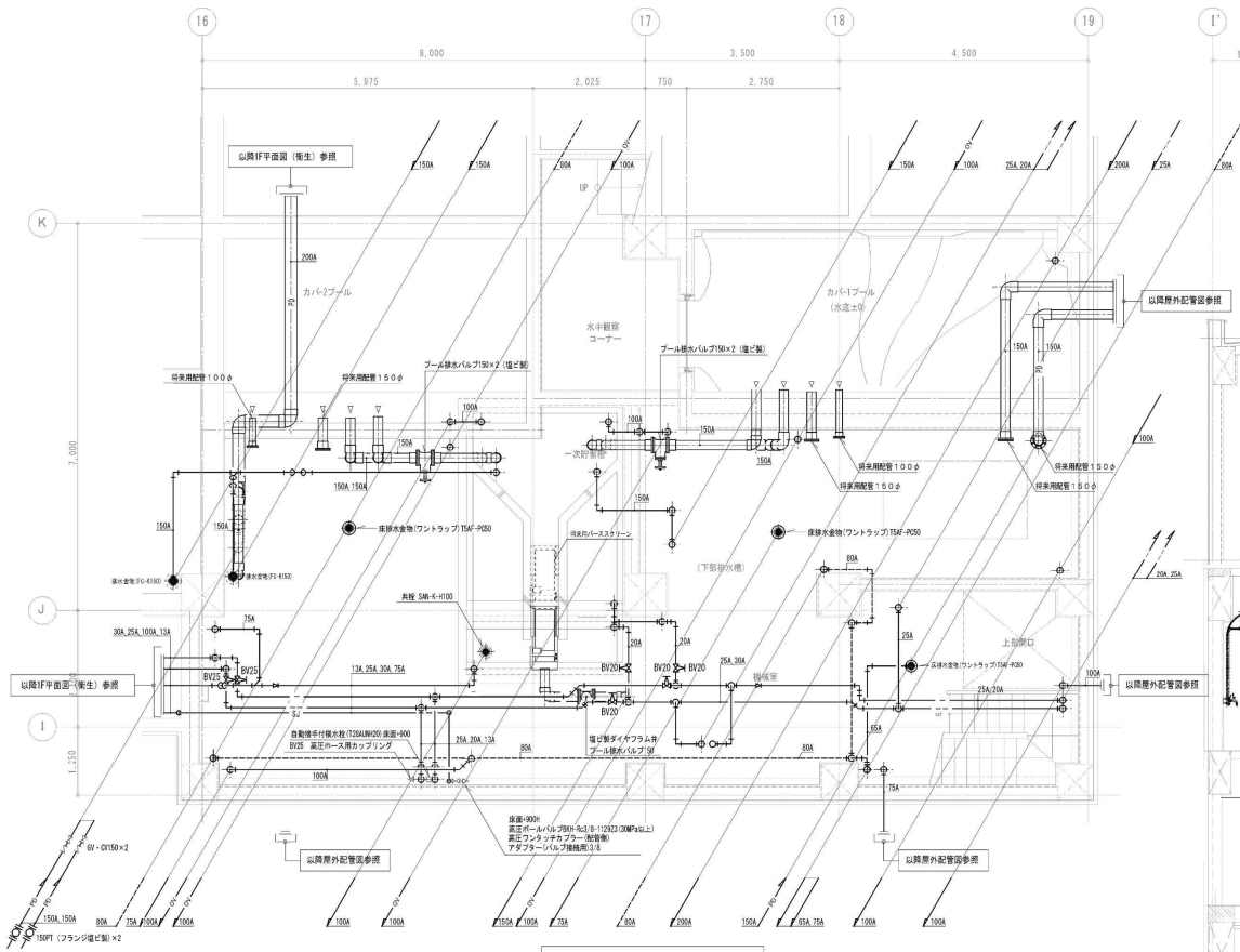
地階機械室 平面図 S=1/50
