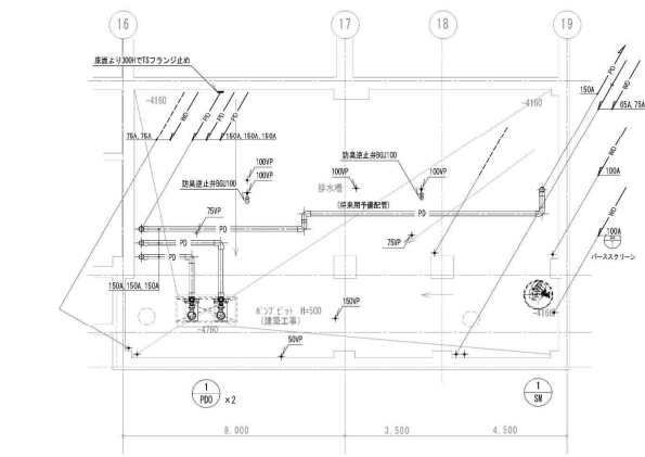
排水槽 平面図 S=1/100
