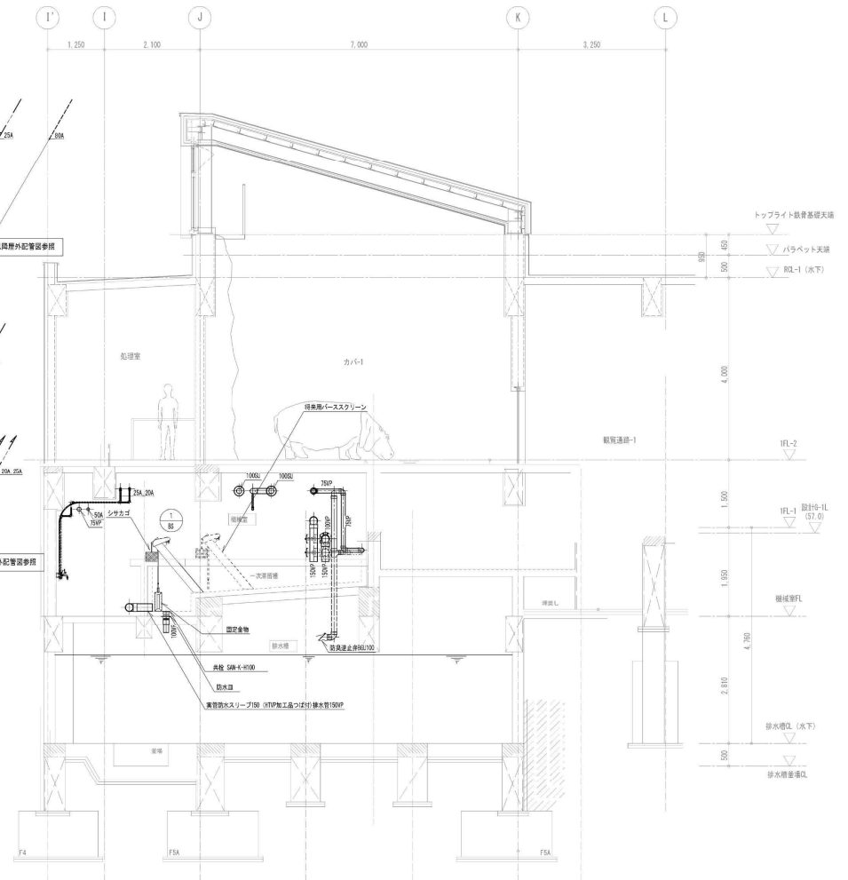
地階機械室 断面図 S=1/50
