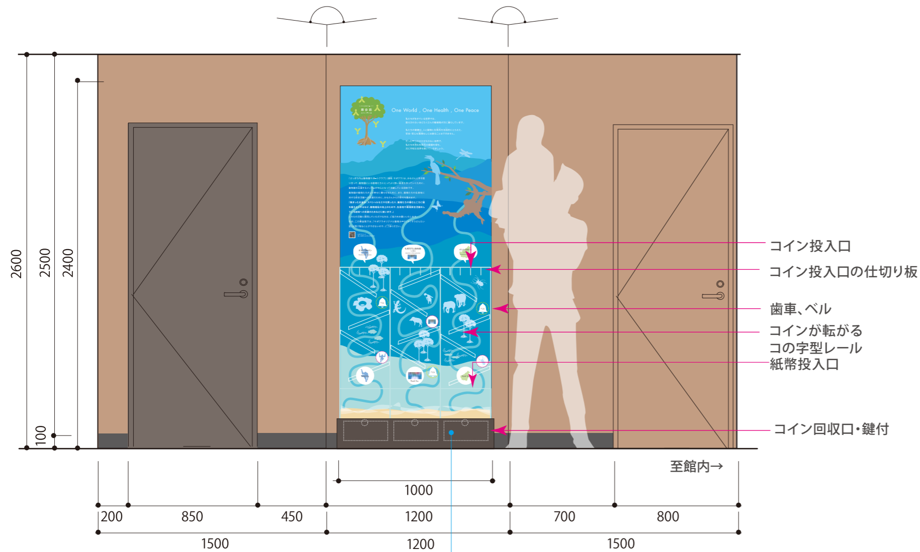
3-02 ①募金箱:W1040*H2400*D200 木造作・インクジェット出力シート貼 (マットラミ加工・巻込み貼)+亚克力ケース加工
