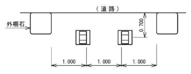
D部詳細図 S=1/00
