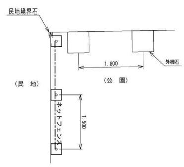
A部詳細図 S=1/00
