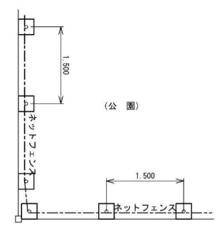
B部詳細図 S=1/00
