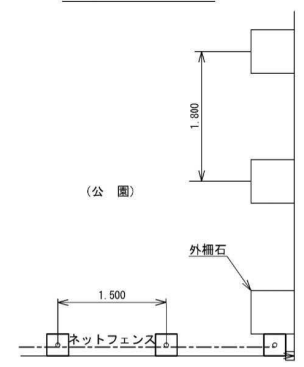
C部詳細図 S=1/00
