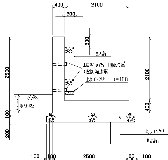
構造図
