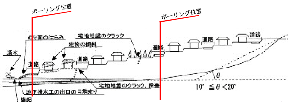
図4-2-2 盛土縦断位置における調査位置選定の考え方
