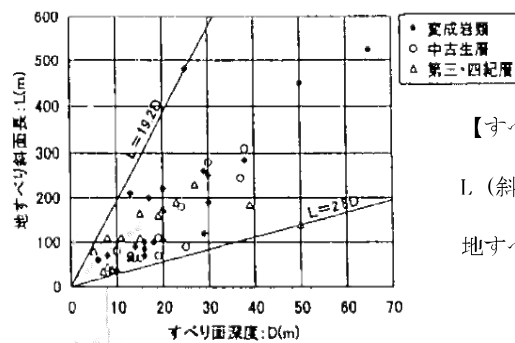
図 6-3-2 すべり面深度に対する地すべり斜面長の関係
