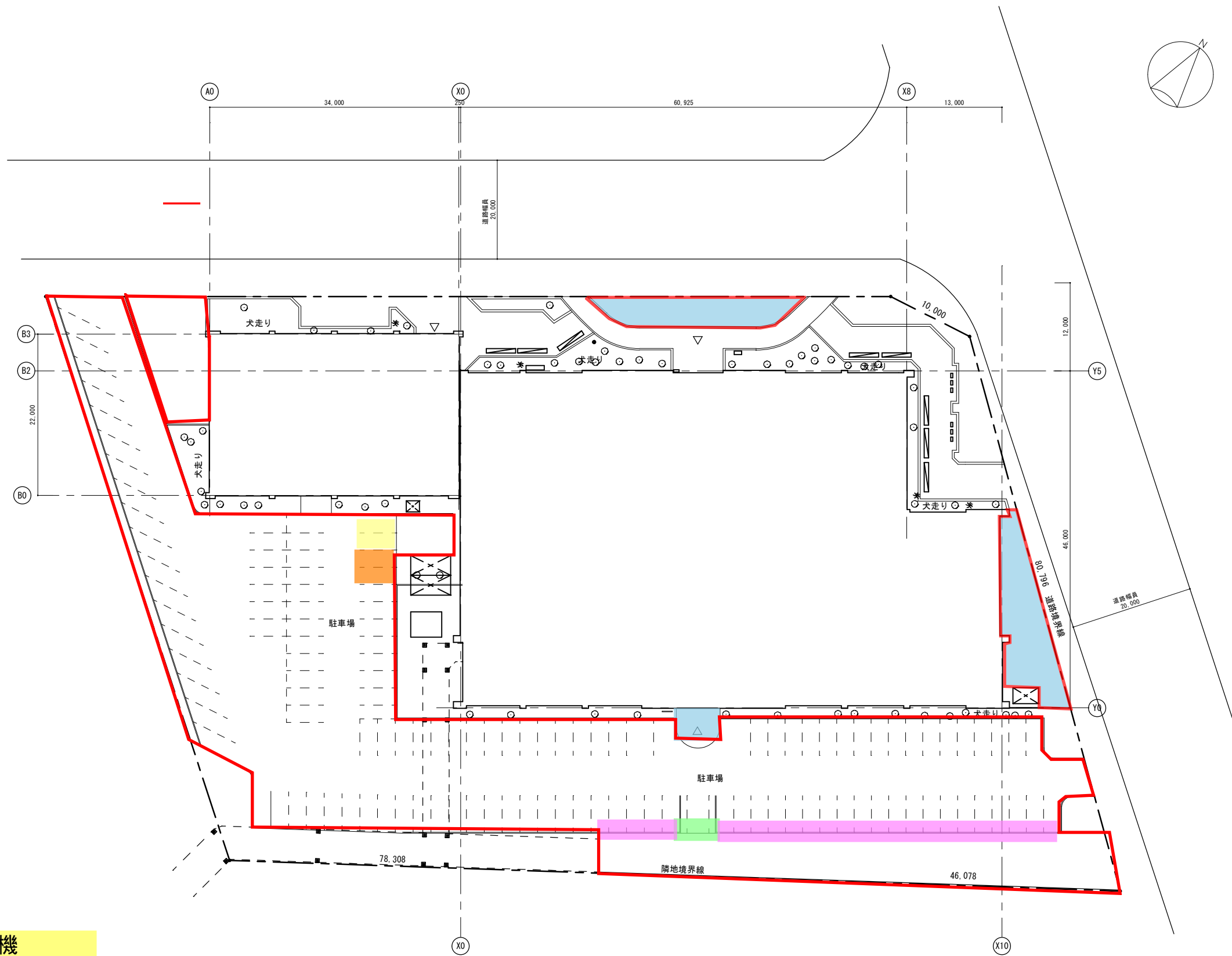
配置図 1/300
