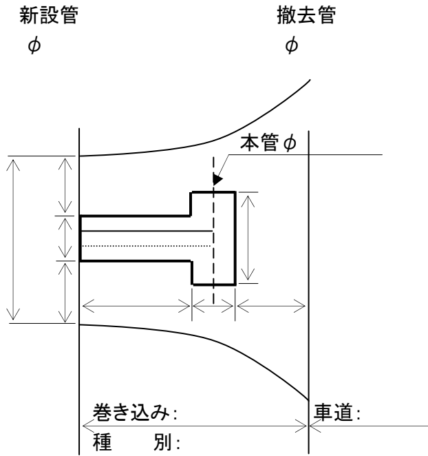
平面図
