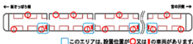
非常通報ボタン車内配置図
