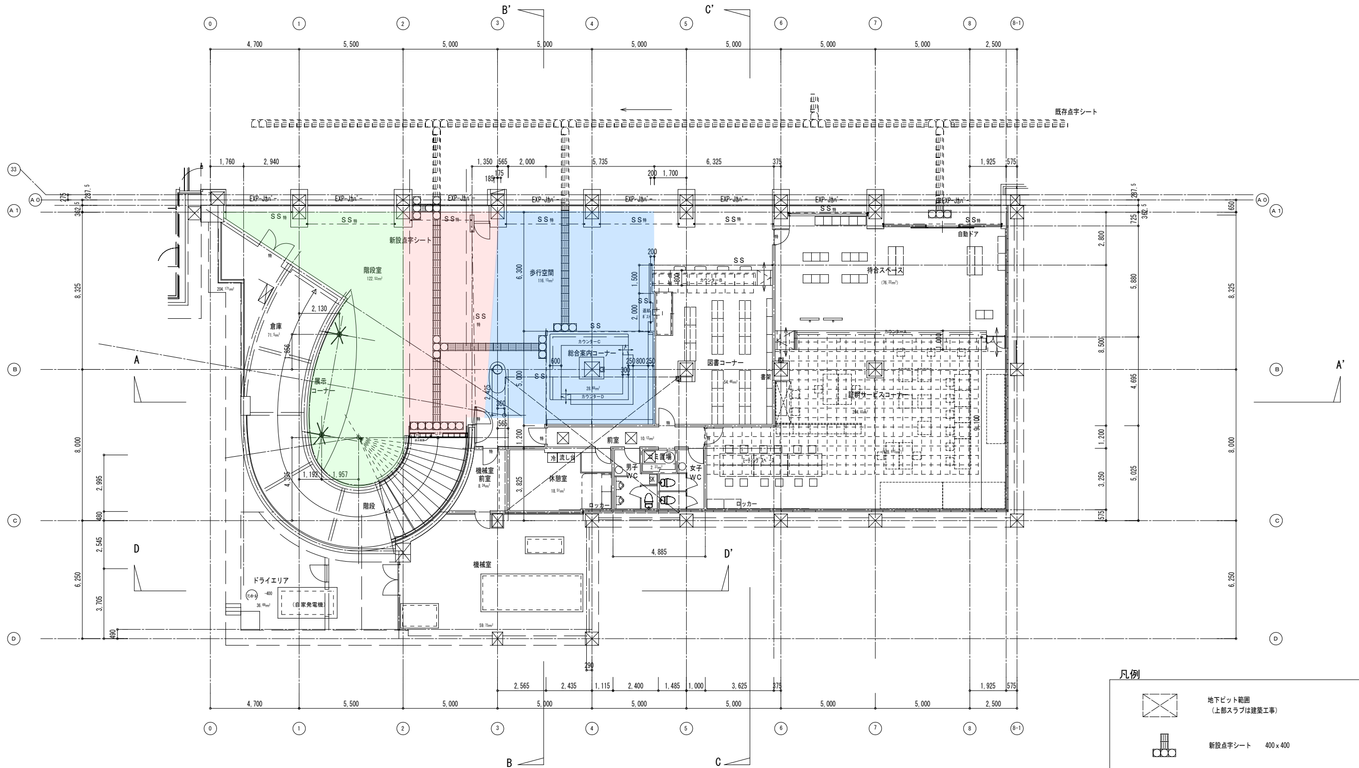
地下1階平面図
