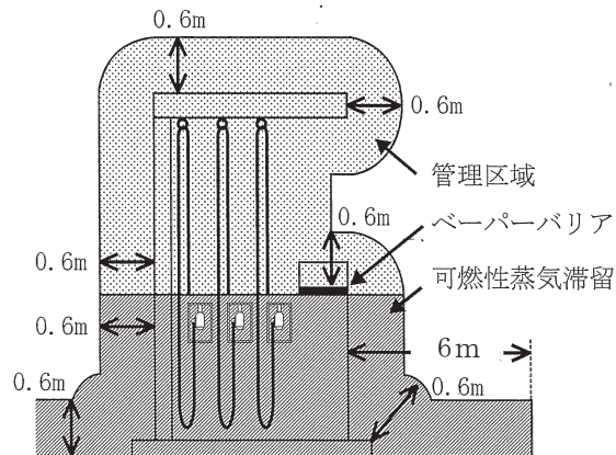
第18－3－4図 地上式固定給油設備（可燃性蒸気流入防止構造）
