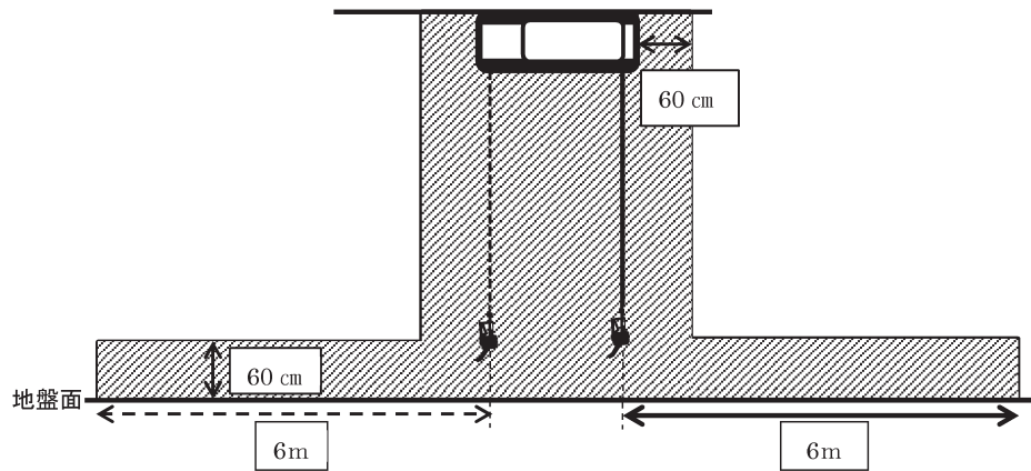
第18－4図 懸垂式固定給油設備
