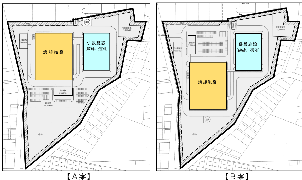
【A案】 【B案】 図 2-4-4 方法書時点の施設配置計画図
