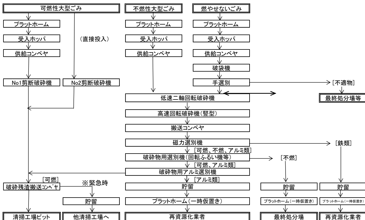
図2-4-8 破碎施設処理フロー(案)
