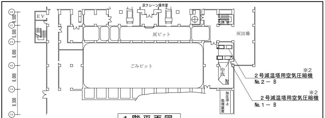
1階平面図
