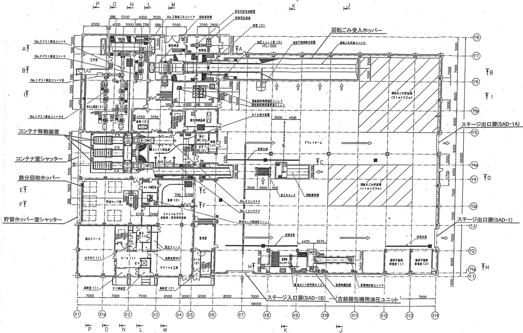
図面名 図番 1階機器配置図 3
